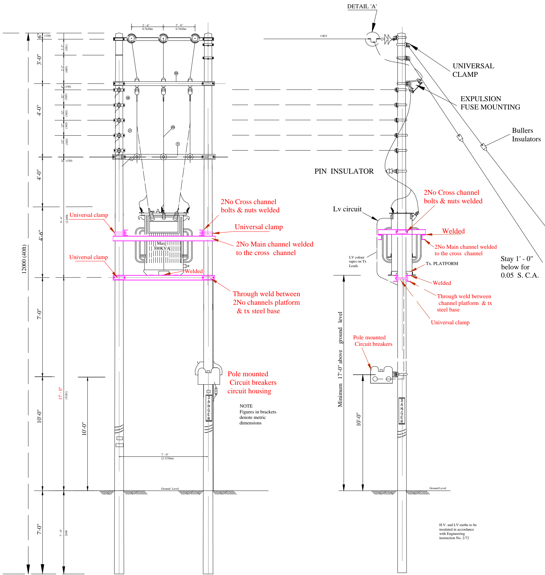
ELEVATION
