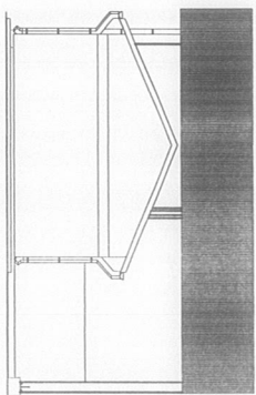
ELEVATION S-2
